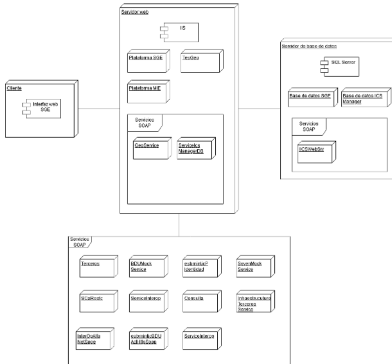
Figura: Diagrama SGE
