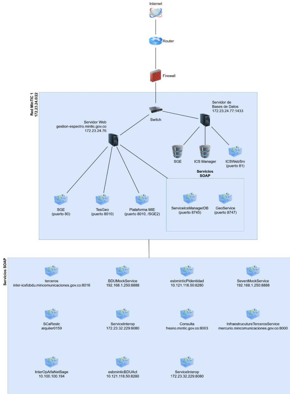
Figura: Despliegue Infraestructura SGE
