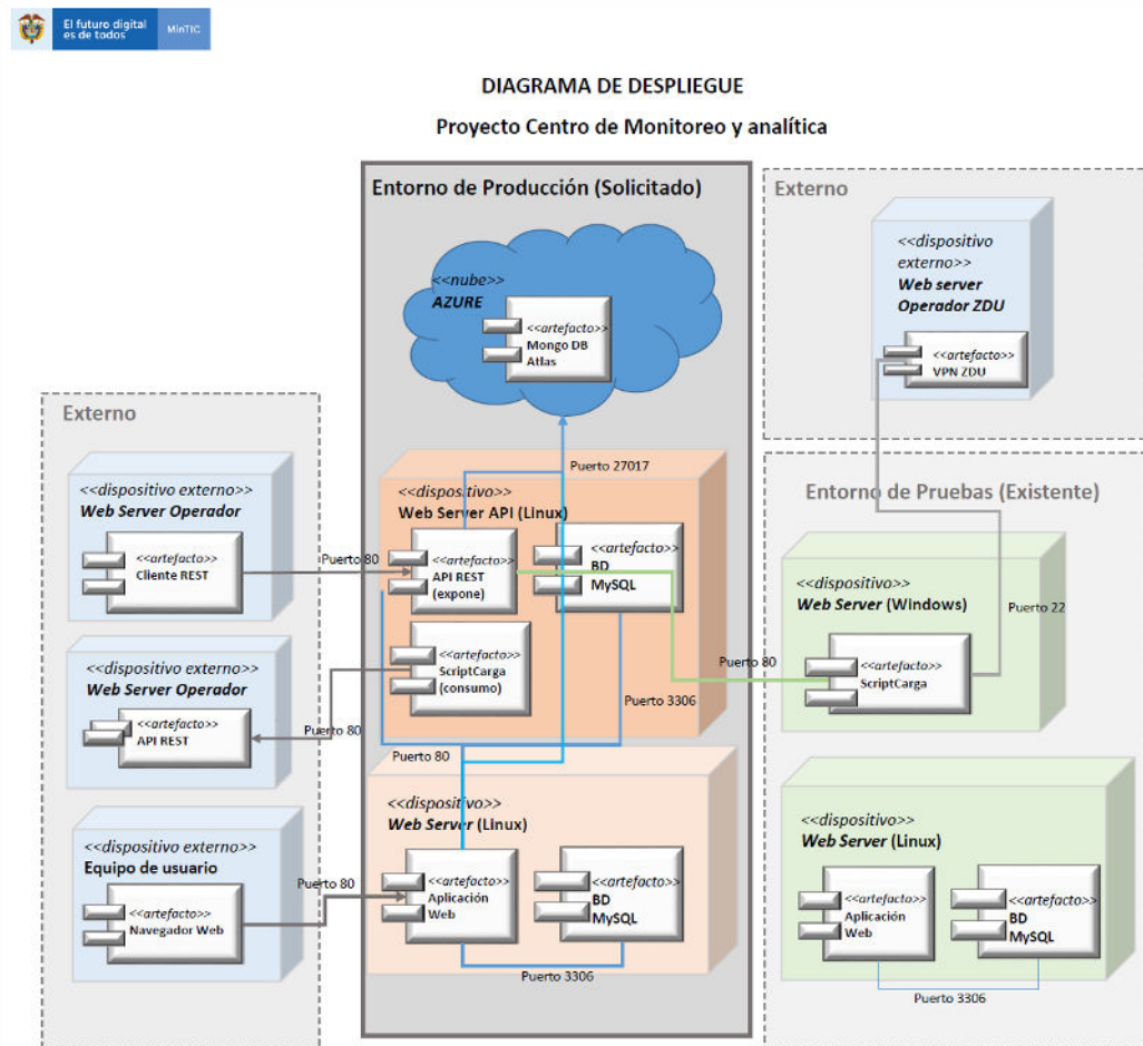
Figura: Diagrama de despliegue DataTIC
